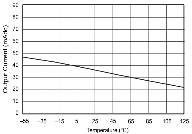
图 6-48. 拉电流限制
