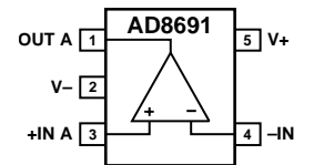
图2. 5引脚SC70
